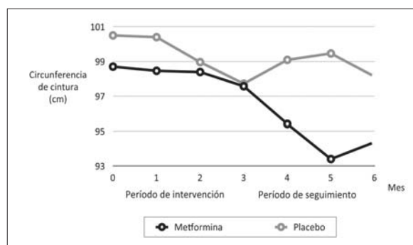
Figura 3. Curva de la circunferencia de cintura a lo largo del estudio.
